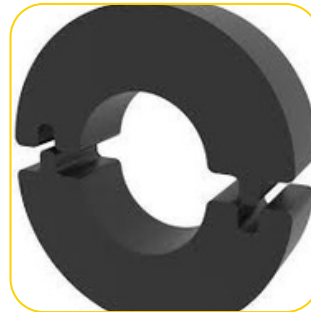
U Strap RSI
