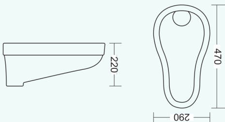
GI-433 | IWC (18\") OPEN RIM
